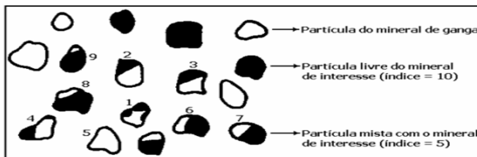
FIGURA 1 - Um exemplo de matriz de partículas mistas e livres usadas no cálculo do grau de liberação (GAUDIN, 1939 a-pud LUZ et al 2010).
