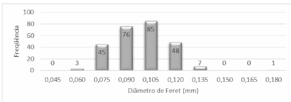
GRÁFICO 5 - Análise granulométrica da malha de 200# (0,074 mm).
