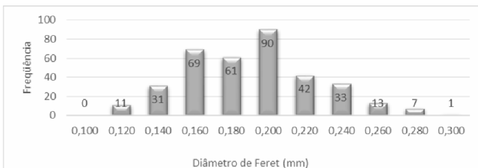
GRÁFICO 3 - Análise granulométrica da malha de 100# (0,149 mm).
