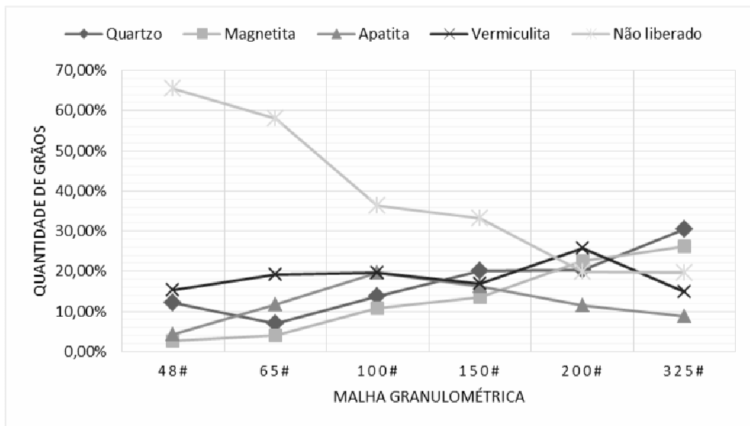
GRÁFICO 7 - Espectro de liberação com a contagem de diferentes tipos de grãos presentes na amostra
