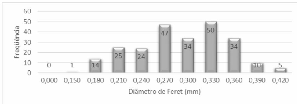
GRÁFICO 2 - Análise granulométrica da malha de 65# (0,210 mm).
