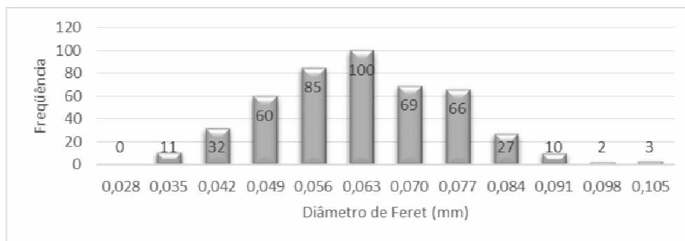
GRÁFICO 6 - Análise granulométrica da malha de 325# (0,044 mm).
