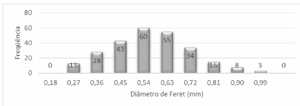
GRÁFICO 1 - Análise Granulométrica da malha de 48# (0,297 mm).
