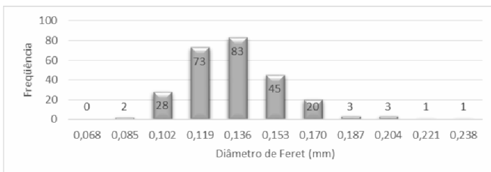
GRÁFICO 4 - Análise granulométrica da malha de 150# (0,105 mm).
